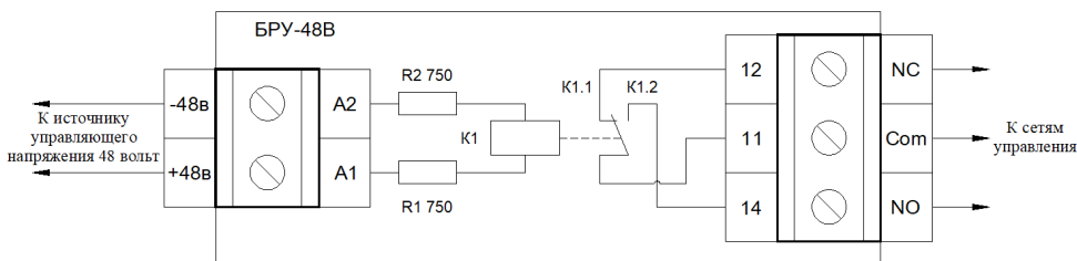
Рис. 1 Схема БРУ-48В
